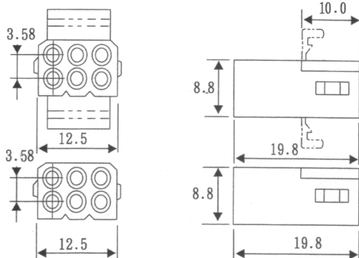
PART NO: H6655-09, 6655E-09
