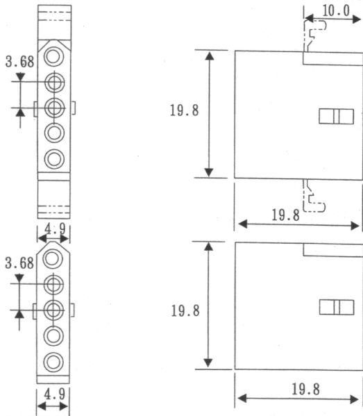
PART NO: H6655-06, 6655E-06
