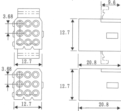
PART NO: H6655-09, 6655E-09
