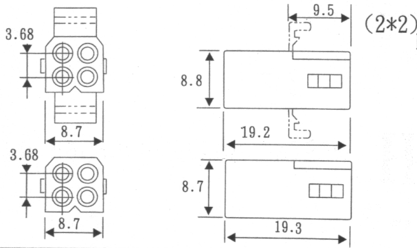
PART NO: H6655-05, 6655E-05
