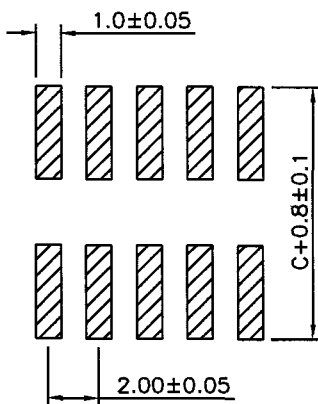
P.C.B LAYOUT
